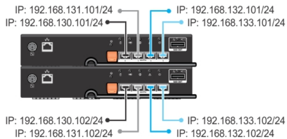
Ilustración 1. Ocho hosts con una única ruta de datos
